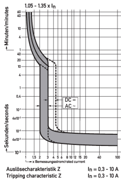
Diagramas Interruptores magnetotérmicos DLS 6i Z0,3-2
