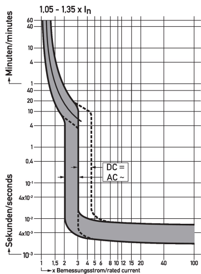
Kennlinie Char. Z
