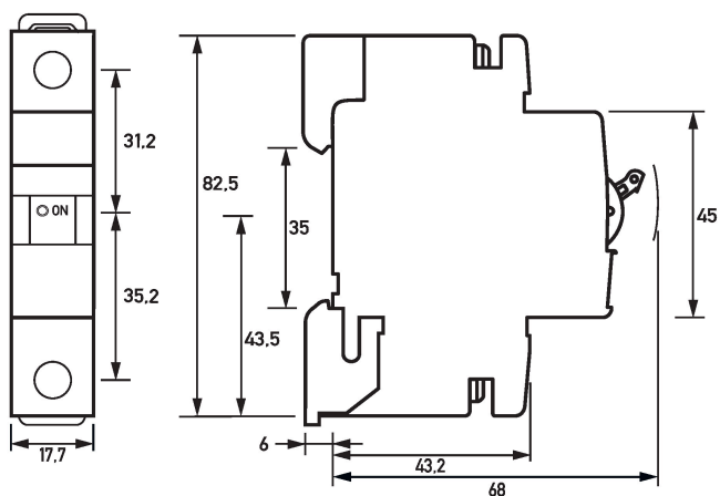
Maßzeichnung DLS 6i, Z-Charakteristik, einpolig, 10kA (Gruppenansicht)
