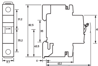
Maßzeichnung Gruppenansicht
