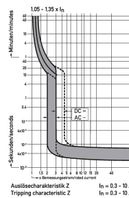
Curva característica Característica Z
