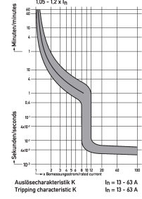
Curva característica Característica K
