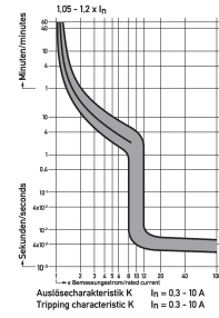
Curva característica Característica K
