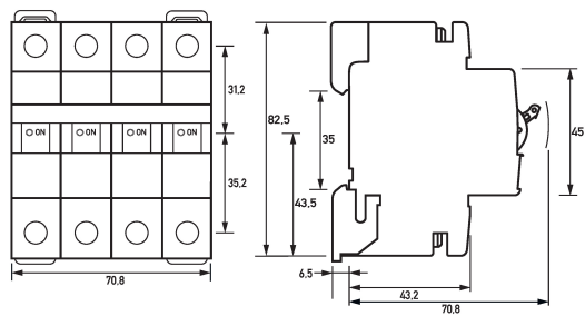
Dibujo acotado Interruptores magnetotérmicos DLS 6i K13-3+N
