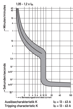
Diagramas Interruptores magnetotérmicos DLS 6i K13-3+N
