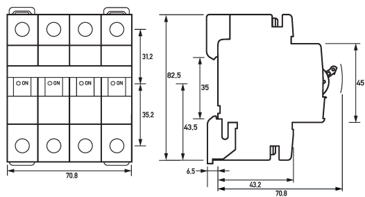
Dibujo acotado Interruptores magnetotérmicos DLS 6i K5-3+N
