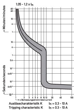
Diagramas Interruptores magnetotérmicos DLS 6i K5-3+N
