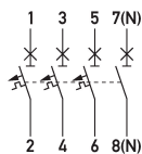
Ejemplo de cableado Interruptores magnetotérmicos DLS 6i K5-3+N
