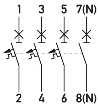
Anschlussschema DLS 6i, K-Charakteristik, dreipolig+N, 10kA
