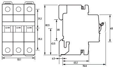
Dibujo acotado Vista de grupos
