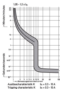
Diagramme Leitungsschutzschalter DLS 6i Ko6-3
