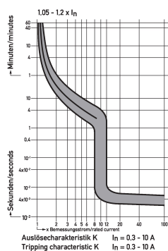
Diagramme Leitungsschutzschalter DLS 6i K4-3
