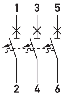
Anschlusschema DLS 6i, K-Charakteristik, dreipolig, 10kA
