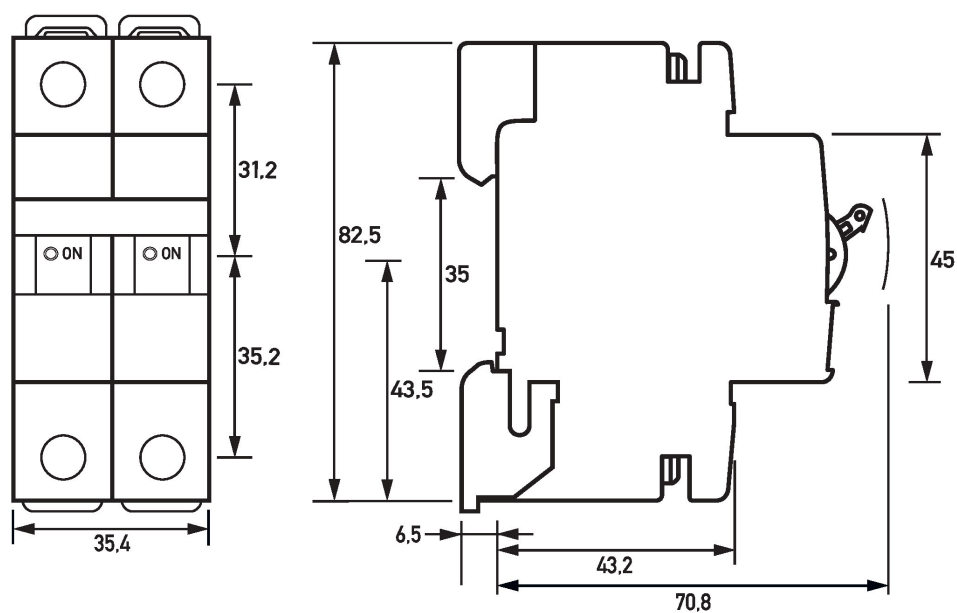
Dibujo acotado DLS 6i, característica K, dos polos, 10kA (Vista de grupos)
