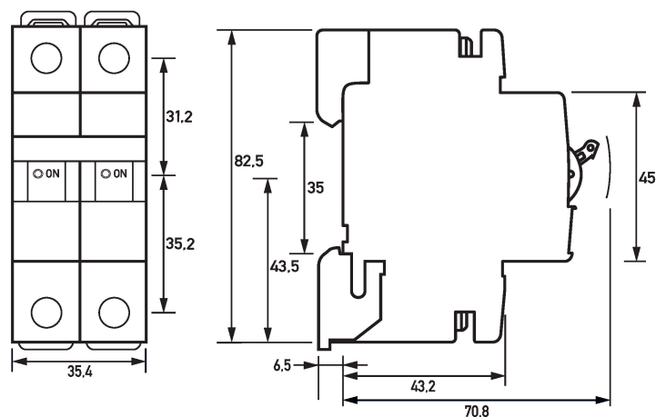
Maßzeichnung DLS 6i, K-Charakteristik, zweipolig, 10kA (Gruppenansicht)
