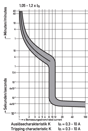
Curva característica Característica K
