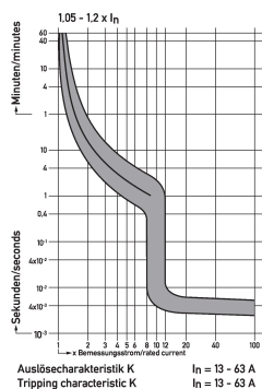
Diagramme Leitungsschutzschalter DLS 6i K50-1
