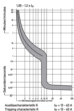
Diagramme Leitungsschutzschalter DLS 6i K32-1
