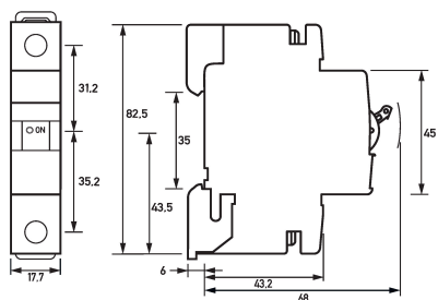
Maßzeichnung Leitungsschutzschalter DLS 6i K32-1
