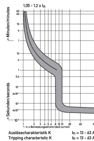
Curva característica Característica K
