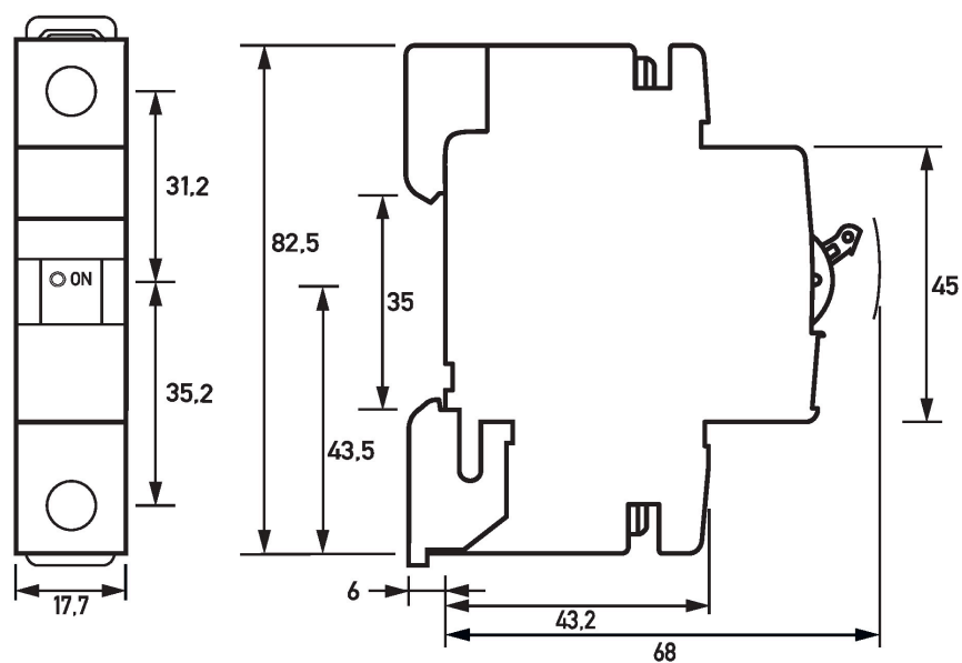
Dibujo acotado DLS 6i, característica K, un polo, 10kA (Vista de grupos)
