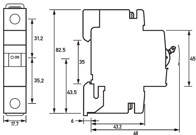
Maßzeichnung DLS 6i, K-Charakteristik, einpolig, 10kA (Gruppenansicht)
