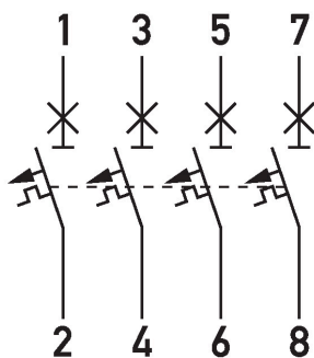
Esquema de conexiones DLS 6i, característica D, cuatro polos, 10kA
