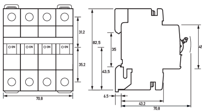
Maßzeichnung Gruppenansicht
