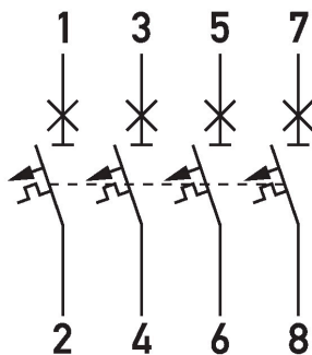
Anschlusschema DLS 6i, D-Charakteristik, vierpolig, 10kA
