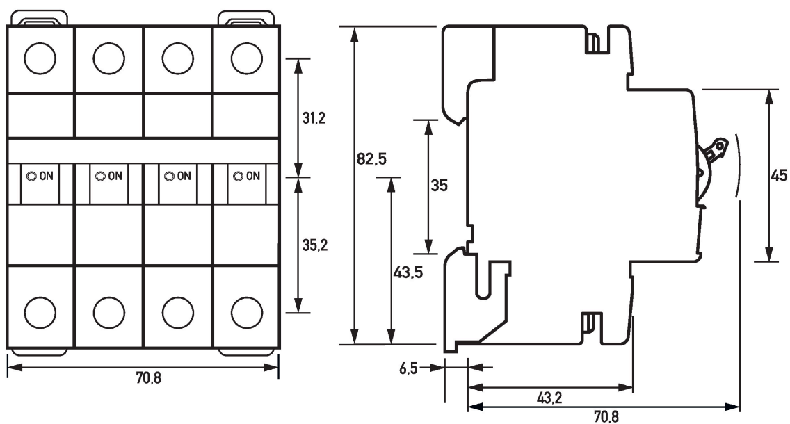
Maßzeichnung DLS 6i, D-Charakteristik, vierpolig, 10kA (Gruppenansicht)
