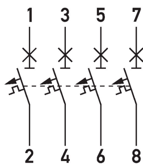
Anschlussschema DLS 6i, D-Charakteristik, vierpolig, 10kA
