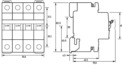
Dibujo acotado Vista de grupos
