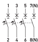
Schaltungsbeispiel Leitungsschutzschalter DLS 6i D20-3+N
