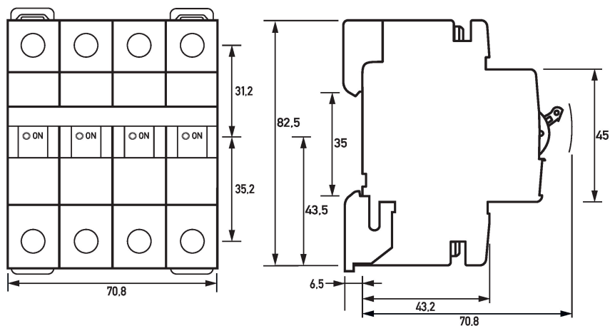
Dibujo acotado DLS 6i, característica D, tres polos+N, 10kA (Vista de grupos)
