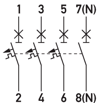
Esquema de conexiones DLS 6i, característica D, tres polos+N, 10kA
