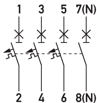
Anschlussschema DLS 6i, D-Charakteristik, dreipolig+N, 10kA
