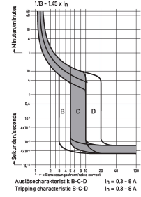
Curva característica Característica B, C, D
