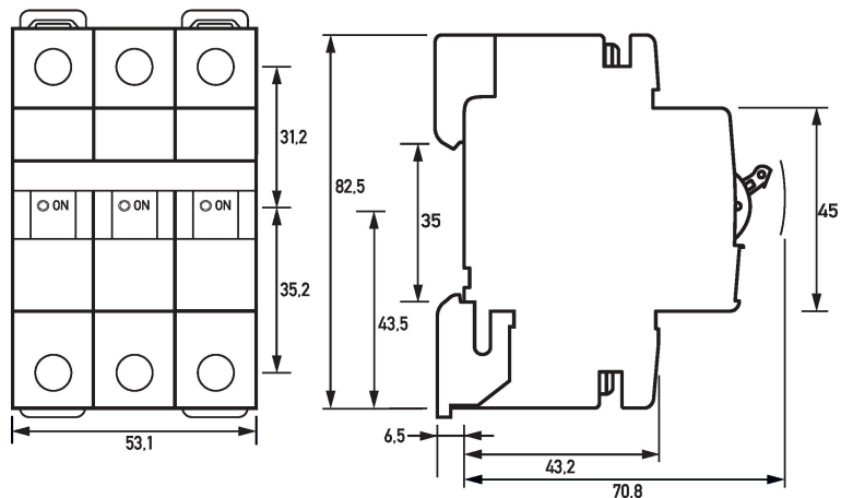
Dibujo acotado DLS 6i, característica D, tres polos, 10kA (Vista de grupos)
