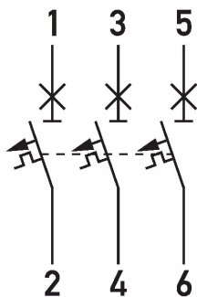
Esquema de conexiones DLS 6i, característica D, tres polos, 10kA
