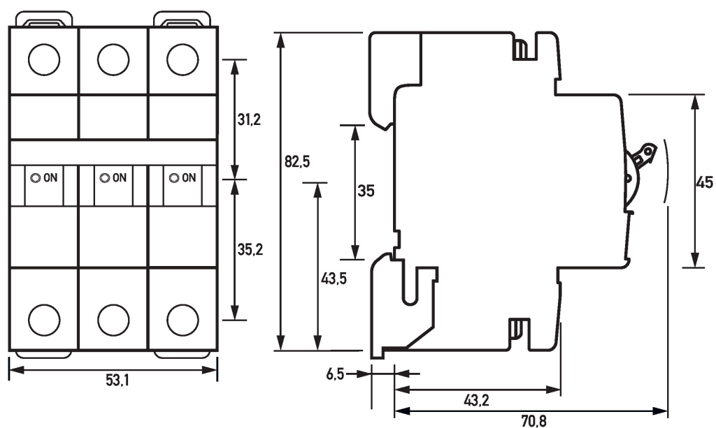
Maßzeichnung DLS 6i, D-Charakteristik, dreipolig, 10kA (Gruppenansicht)
