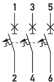
Anschlussschema DLS 6i, D-Charakteristik, dreipolig, 10kA
