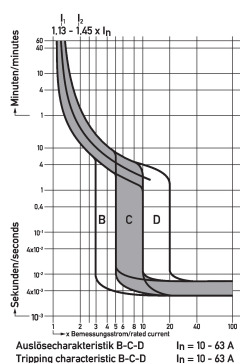
Diagramme Leitungsschutzschalter DLS 6i D63-2
