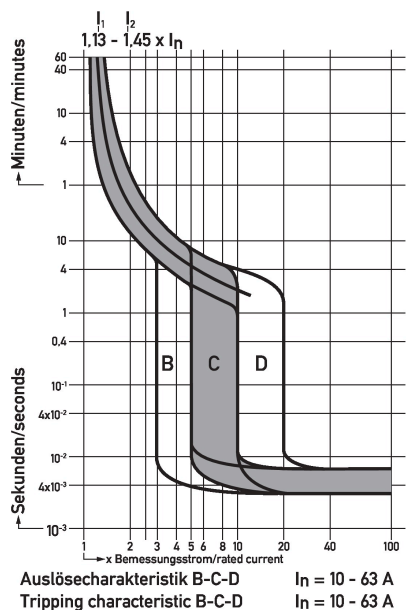
Curva característica Característica B, C, D
