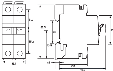
Dibujo acotado Interruptores magnetotérmicos DLS 6i D16-2
