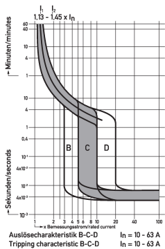
Diagramas Interruptores magnetotérmicos DLS 6i D16-2
