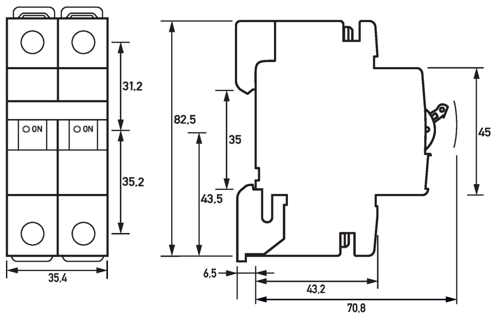
Maßzeichnung DLS 6i, D-Charakteristik, zweipolig, 10kA (Gruppenansicht)
