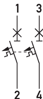
Esquema de conexiones DLS 6i, característica D, dos polos, 10kA
