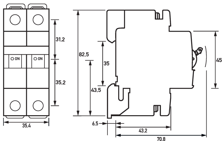
Dibujo acotado DLS 6i, característica D, dos polos, 10kA (Vista de grupos)
