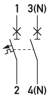
Anschlussschema DLS 6i, D-Charakteristik, einpolig+N, 10kA
