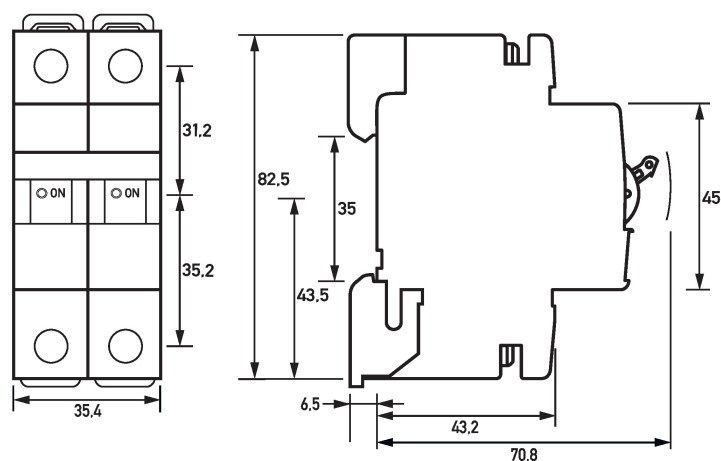
Maßzeichnung DLS 6i, D-Charakteristik, einpolig+N, 10kA (Gruppenansicht)
