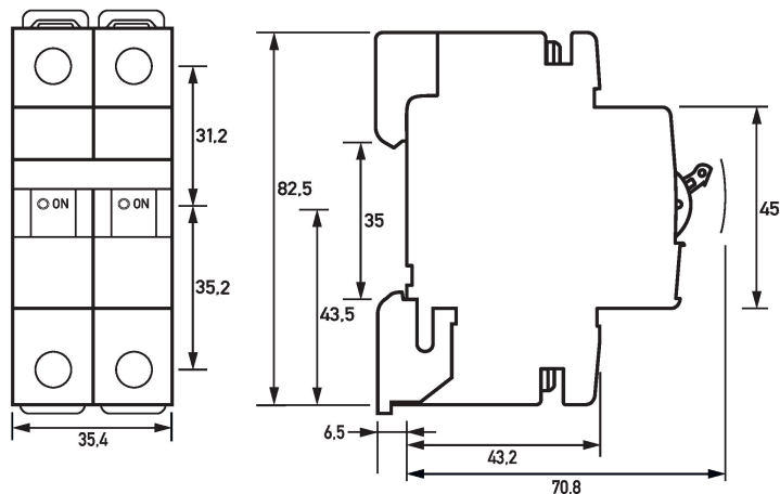
Dibujo acotado DLS 6i, característica D, un polo+N, 10kA (Vista de grupos)
