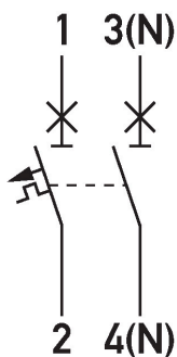
Esquema de conexiones DLS 6i, característica D, un polo+N, 10kA
