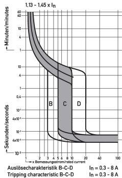
Diagramas Interruptores magnetotérmicos DLS 6i Do4-1
