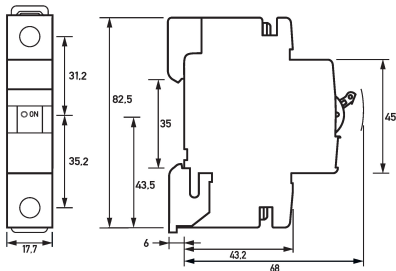
Dibujo acotado Interruptores magnetotérmicos DLS 6i Do4-1
