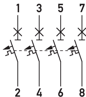
Anschlusschema DLS 6i, C-Charakteristik, vierpolig, 10kA
