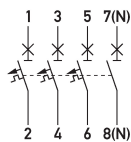
Ejemplo de cableado Interruptores magnetotérmicos DLS 6i C40-3+N
