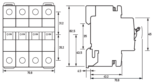
Dibujo acotado Interruptores magnetotérmicos DLS 6i C40-3+N
