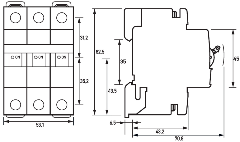
Maßzeichnung DLS 6i, C-Charakteristik, dreipolig, 10kA (Gruppenansicht)
