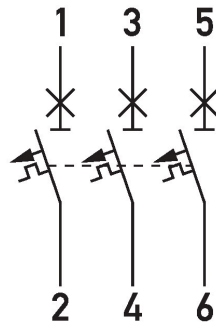
Anschlusschema DLS 6i, C-Charakteristik, dreipolig, 10kA
