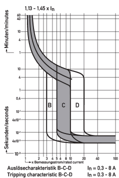
Curva característica Característica B, C, D
