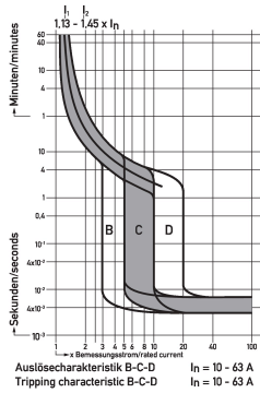
Diagramas Interruptores magnetotérmicos DLS 6i C32-1+N
