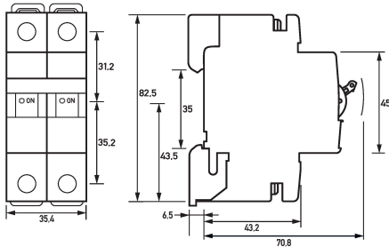
Dibujo acotado Interruptores magnetotérmicos DLS 6i C32-1+N
