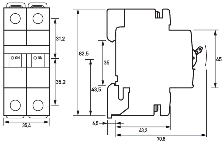
Dibujo acotado Interruptores magnetotérmicos DLS 6i C16-1+N
