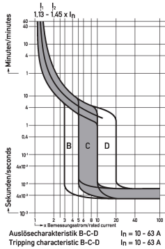
Diagramas Interruptores magnetotérmicos DLS 6i C16-1+N
