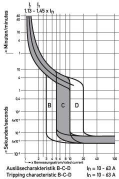
Diagramas Interruptores magnetotérmicos DLS 6i C16-1
