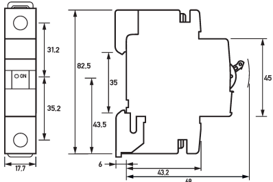
Dibujo acotado Interruptores magnetotérmicos DLS 6i C16-1
