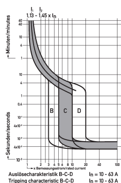
Diagramme Leitungsschutzschalter DLS 6i C16-1
