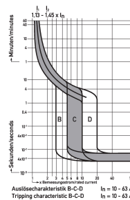
Curva característica Característica B, C, D
